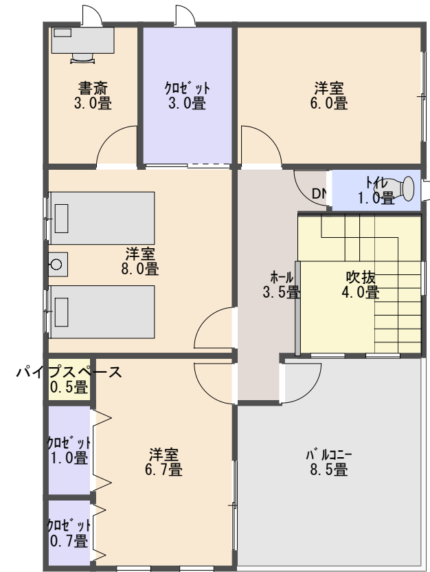
2階 縮尺 1/100
